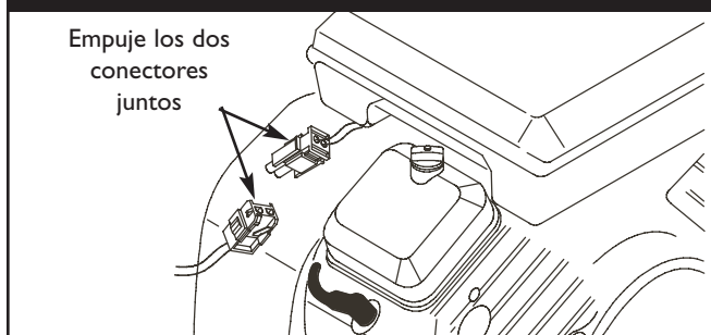
Figura 26 — Conexión del Solenoide de Transferencia de Combustible
